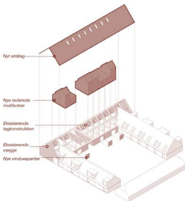
Isometri/ transformation af den store længe med tilføjelse af isolerende multibokse og vinduer
